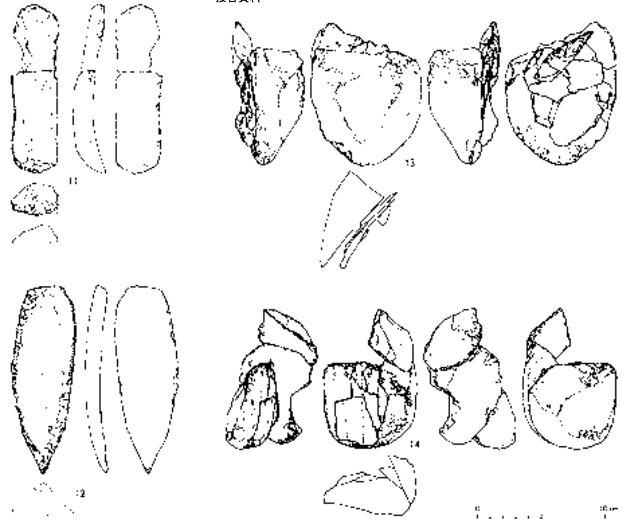
旧白滝 5 遺跡 小型鋸齒縁尖頭器を含む石器群
